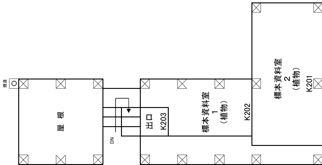
2F 平面図
