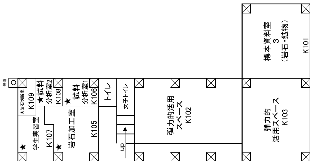
1F 平面図
