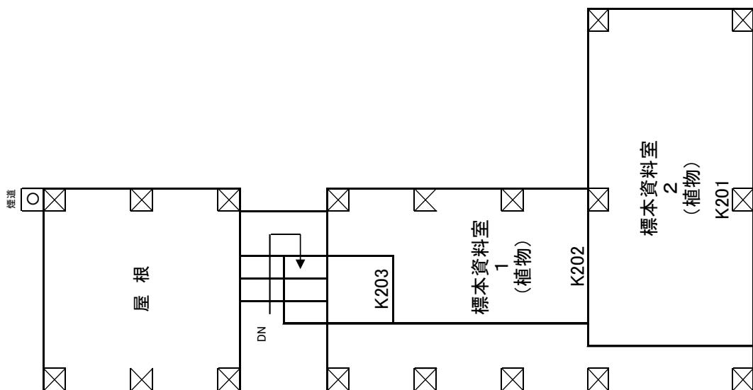
2F 平面図
